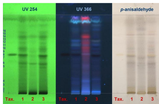
ภาพที่ 1 ที่แอลซีโครมาโทแกรมของสารสกัดเมทานอล (1: สงขลา, 2: ปทุมธานี, 3: สมุทรปราการ) เปรียบเทียบกับสารมาตรฐาน taxifolin (Tax.)
